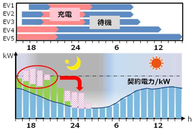
電池残量等の情報から充電タイミングを制御し 契約電力UPを抑制
